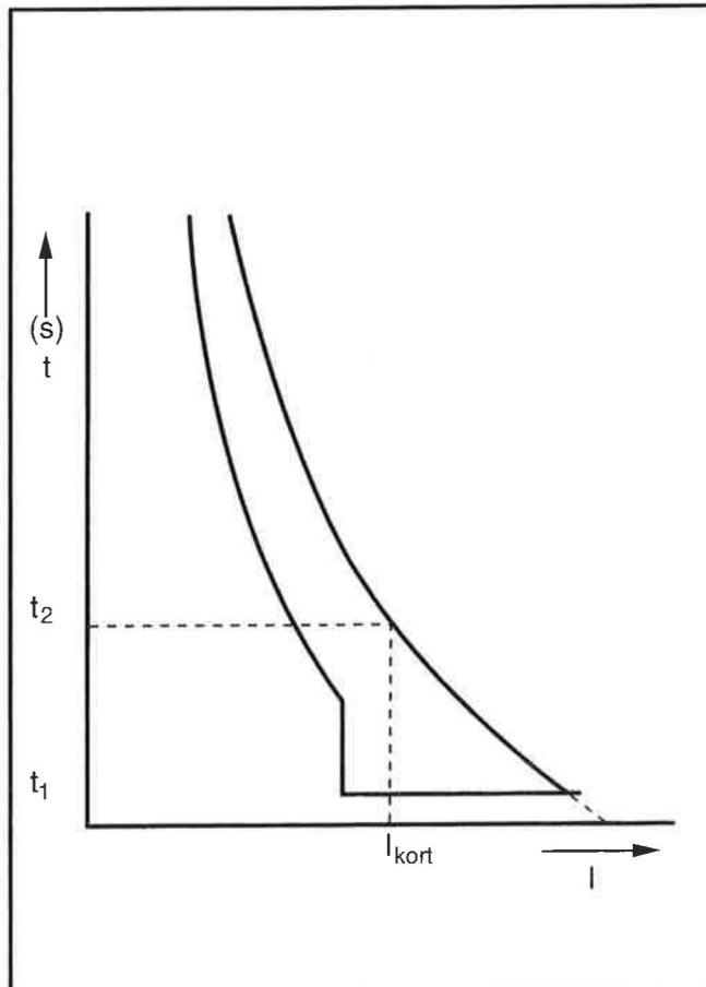
Figuur 14 Controle selectiviteit
