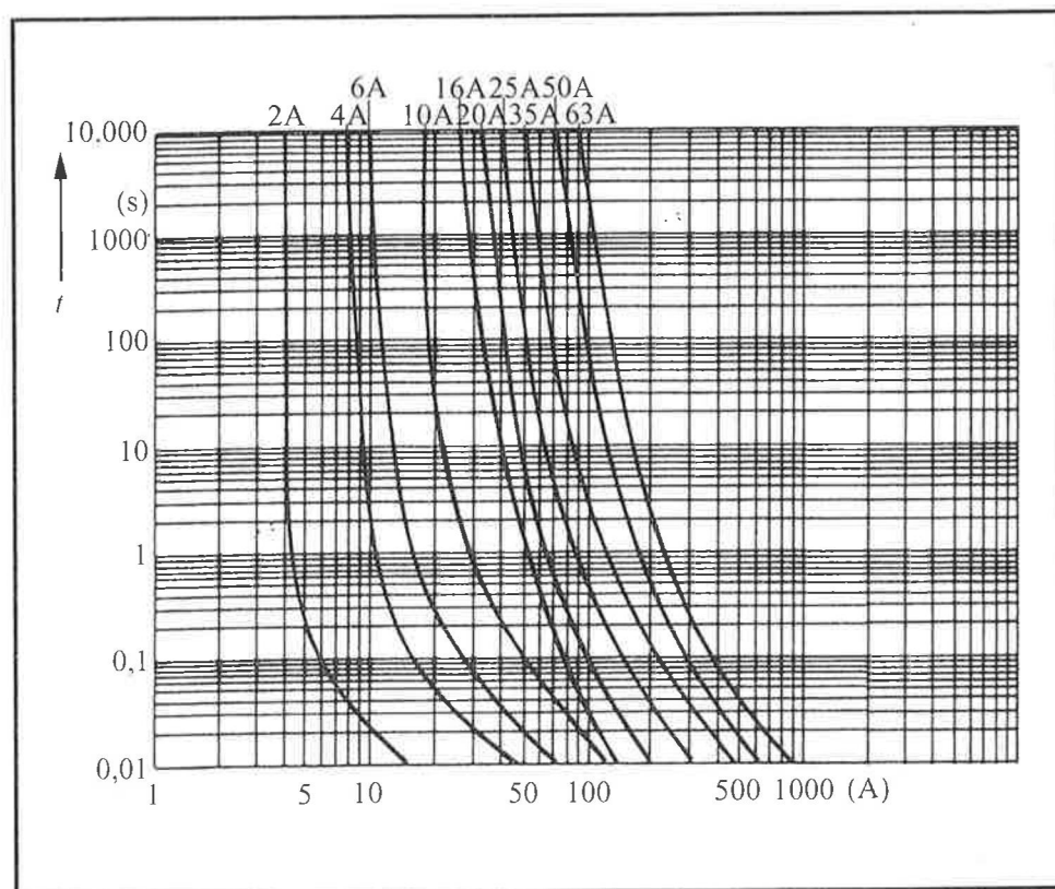
Figuur 11 Smelt- karakteristieken D-patronen (snel)
