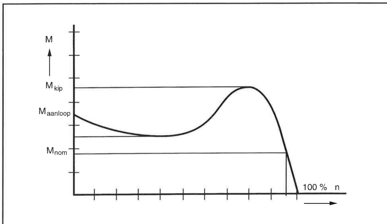
Figuur 2 Koppel-toerenkromme SKA-motor
