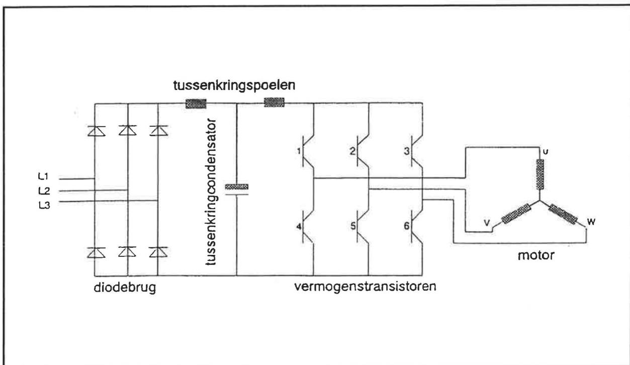
Figuur 7 Het schema van de spanningsbron-frequentie-omzetter
