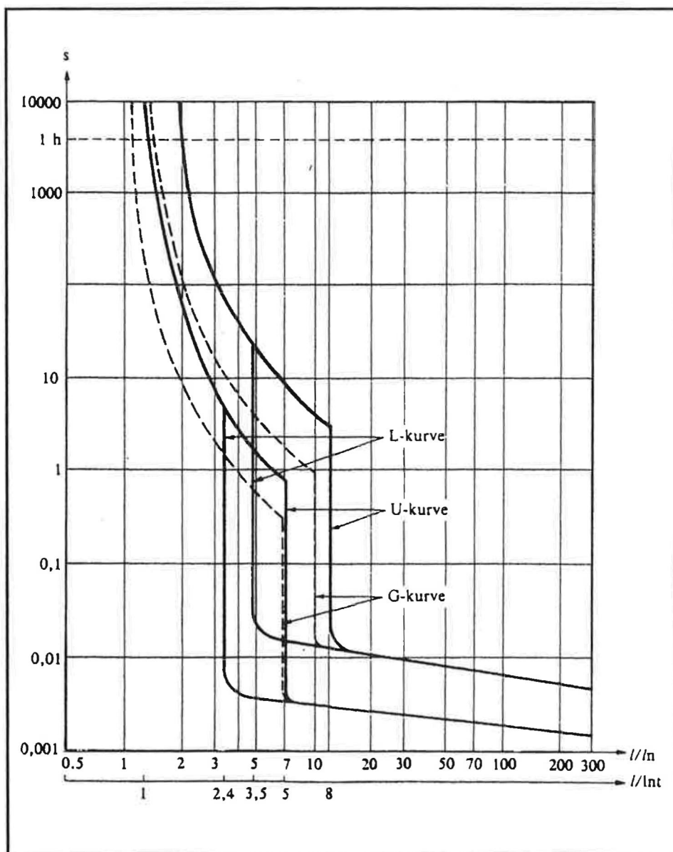
Figuur 13 Uitschakel- karakteristieken automaat
