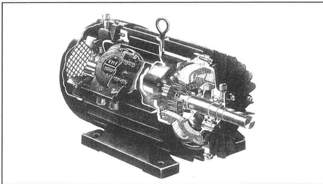
Draaistroommotor
