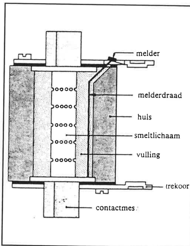
Figuur 9 Doorsnede mespatroon
