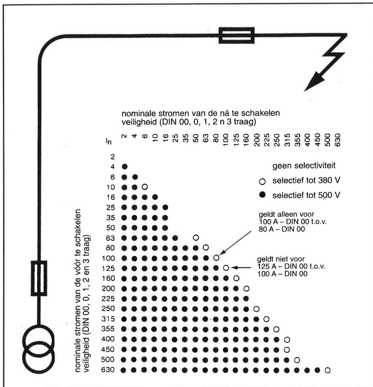
Figuur 16 - Selectiviteit van trage mepatronen DIN-groottes 00, 0, 1, 2 en 3 onder kortsluitomstandigheden
