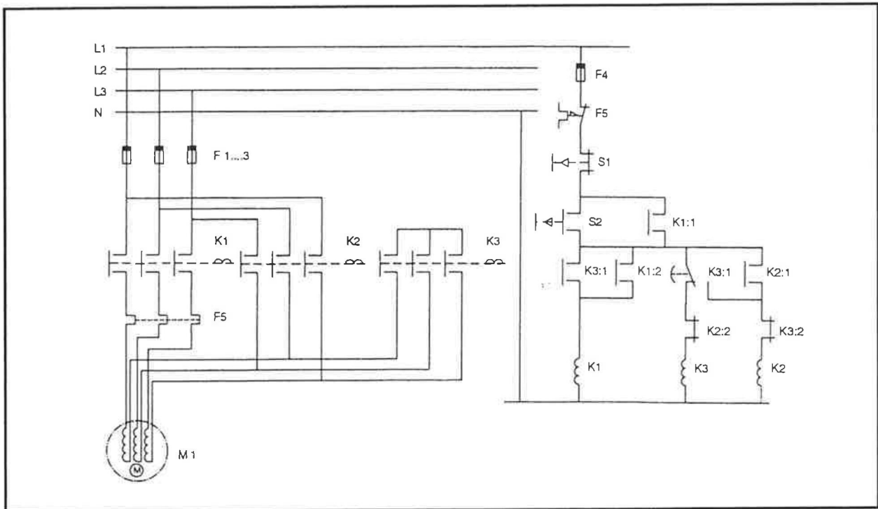
Figuur 5 Draaistroommotor met ster-driehoekaanloop. Hoofdstroom en stuurstroom
