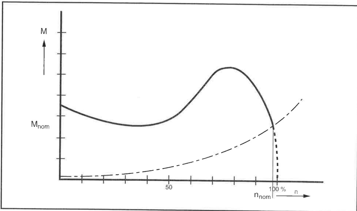
Figuur 4 Koppeldoerenkromme SKA-motor met werktuig
