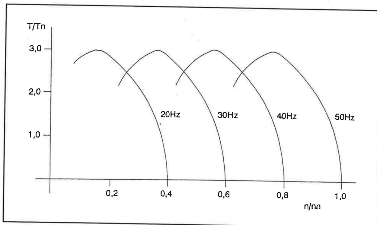
Figuur 6 Koppel-toerendiagram van een SKA in combinatie met een frequentie-omzetter
