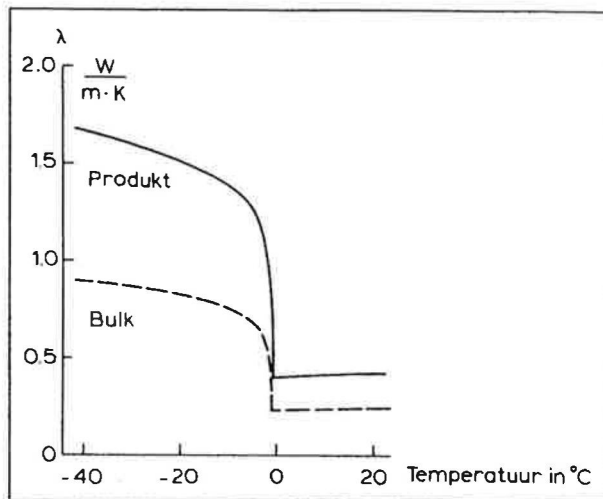
Figuur 2 - Warmtegeleidingscoëfficiënt van appel
