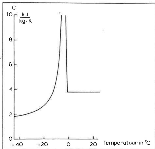
Figuur 1 - Soortelijke warmte van appel
