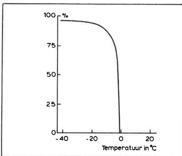
Figuur 3 - Temperatuurvereffeningscoëfficiënt van appel
