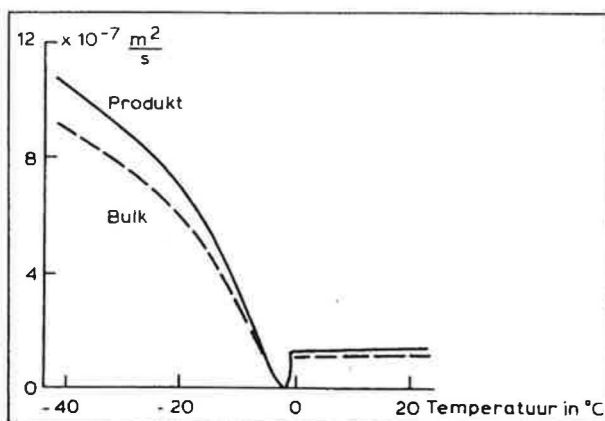
Figuur 3 - Temperatuurvereffeningscoëfficiënt van appel
