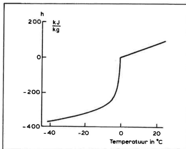
Figuur 4 - Enthalpie van appel
